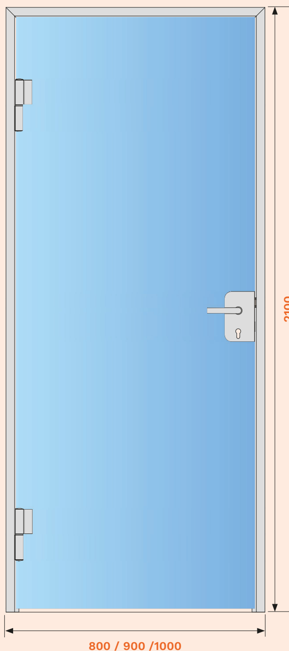
DIN med Evo gångjärn
