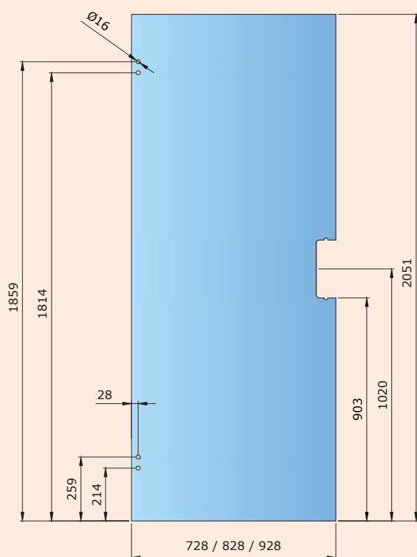
Urtag i glaset för SIS-lås Flexible
