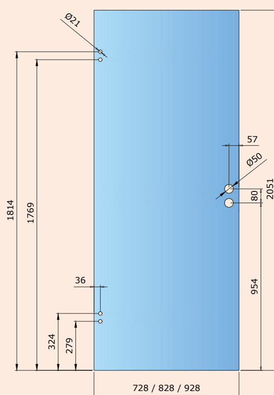
DIN med Evo gångjärn
