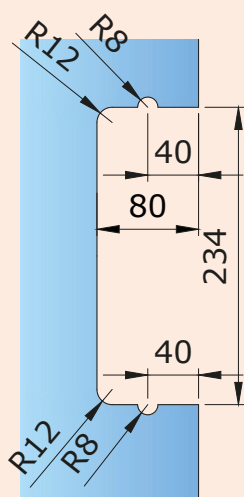
Urtag i glaset för SIS-lås Flexible
