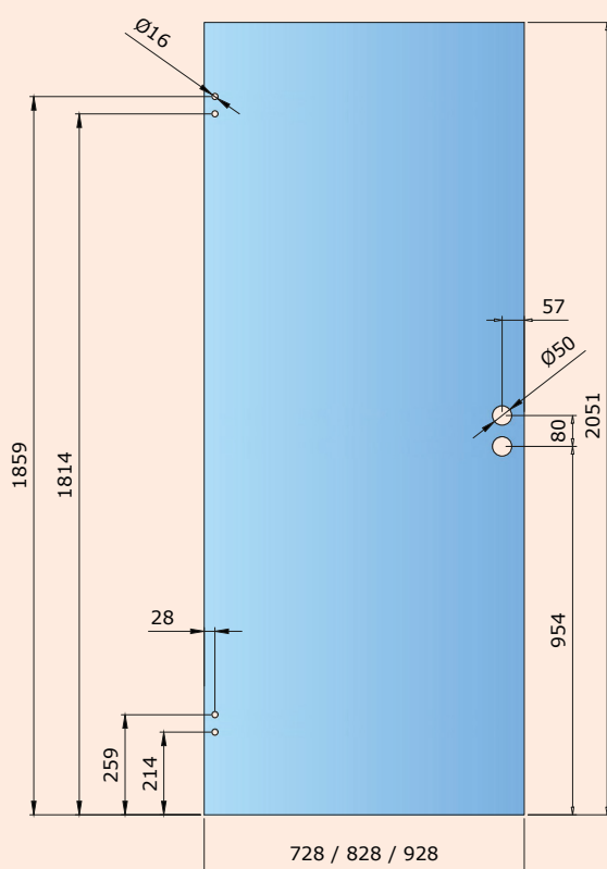
DIN med standard gångjärn
