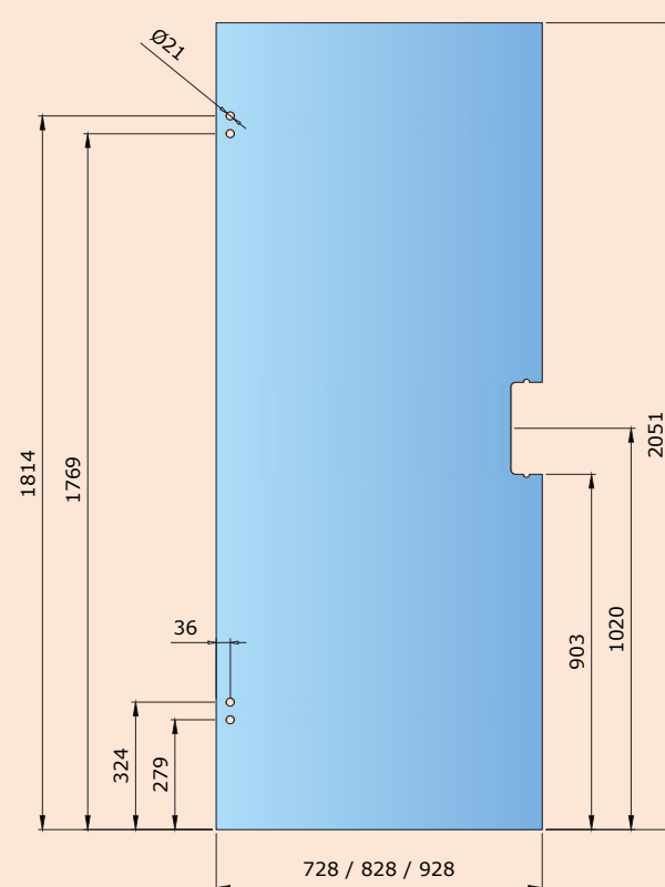
Flexible med 2 st Evo gångjärn
