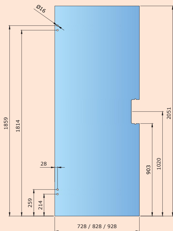
Flexible med standard gångjärn
