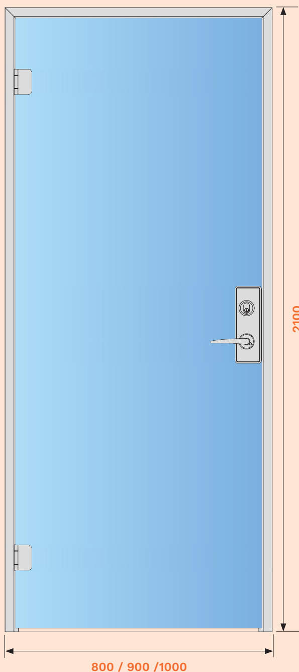
Flexible med standard gångjärn
